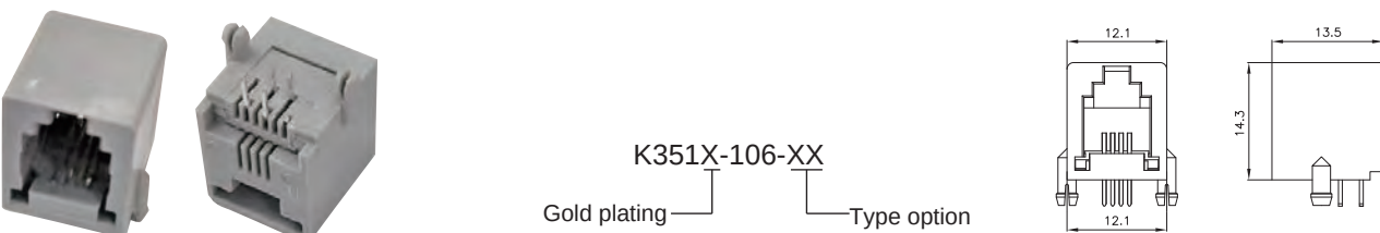
Side Entry Mini L/P 4P PCB Jack
