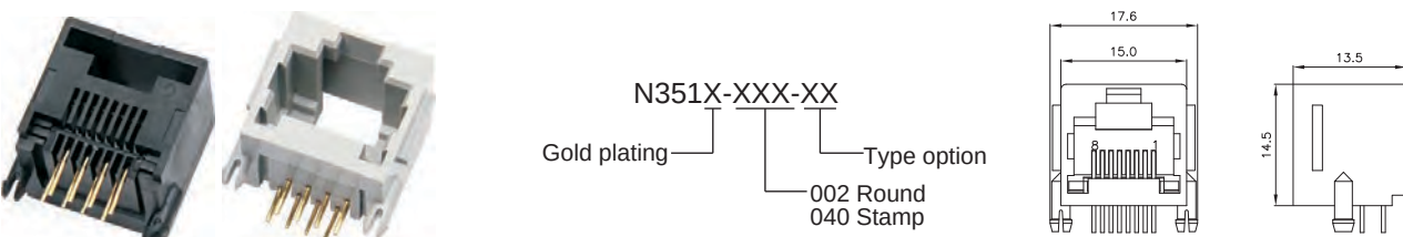
Side Entry Mini L/P 8P PCB Jack
