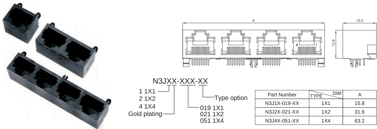
Side Entry 1X1、1X2、1X4 8P Jack UTP (Stamp)
