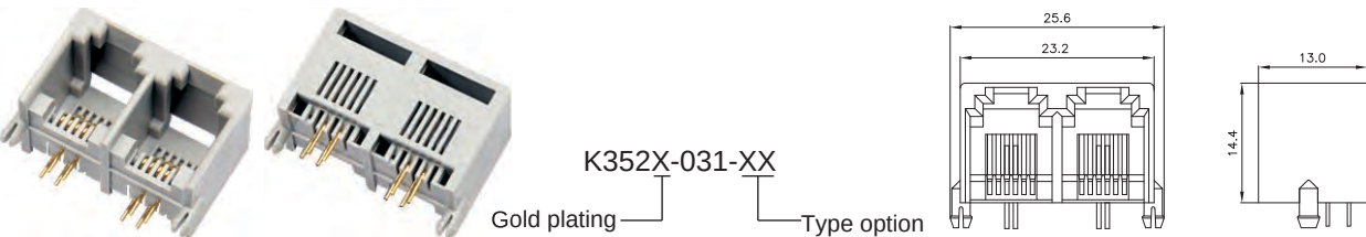
Side Entry Mini L/P 6P PCB Jack
