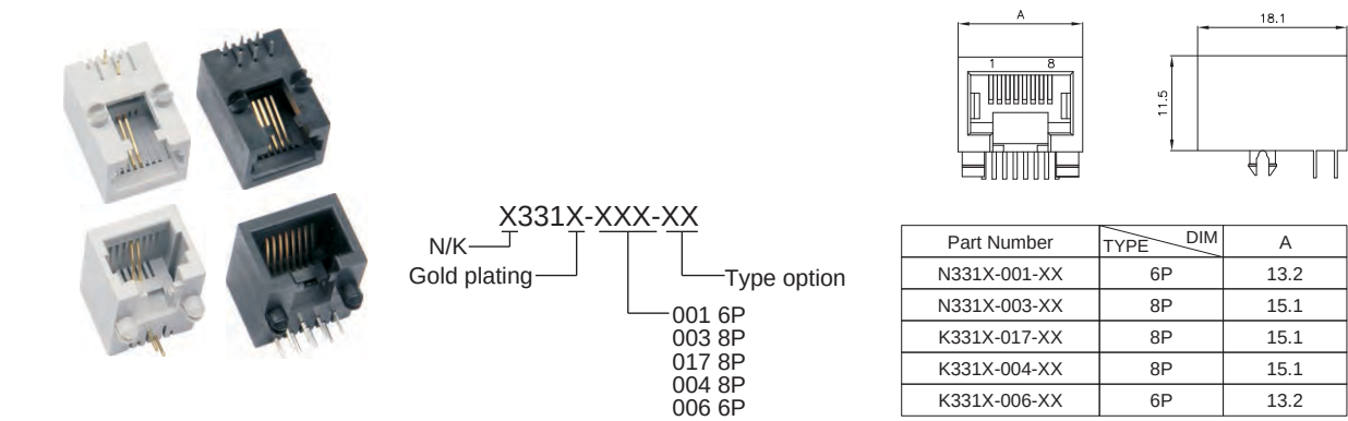
Side Entry 6P 、 8P PCB Jack UTP
