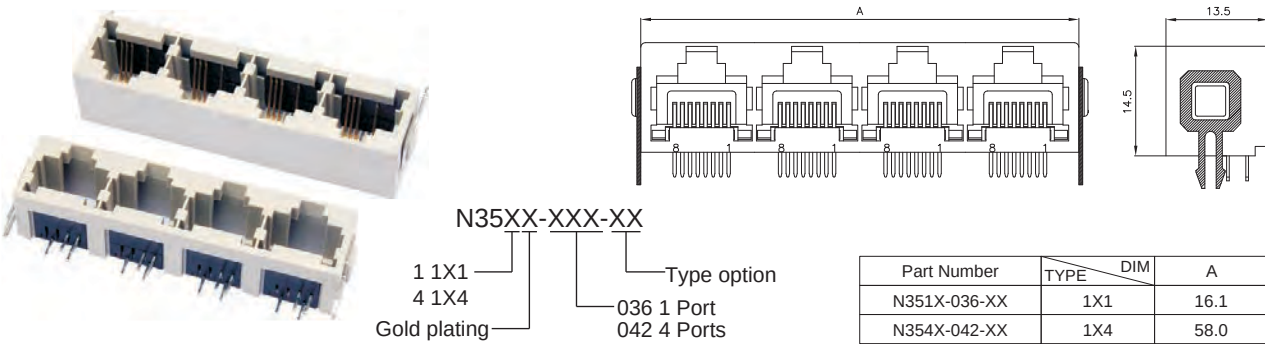
Side Entry Mini L/P 8P STP (Stamp) PCB Jack
