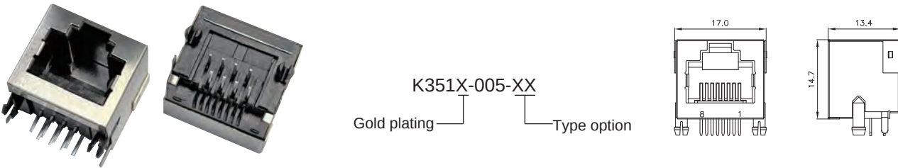
Side Entry Mini L/P 8P PCB Jack
