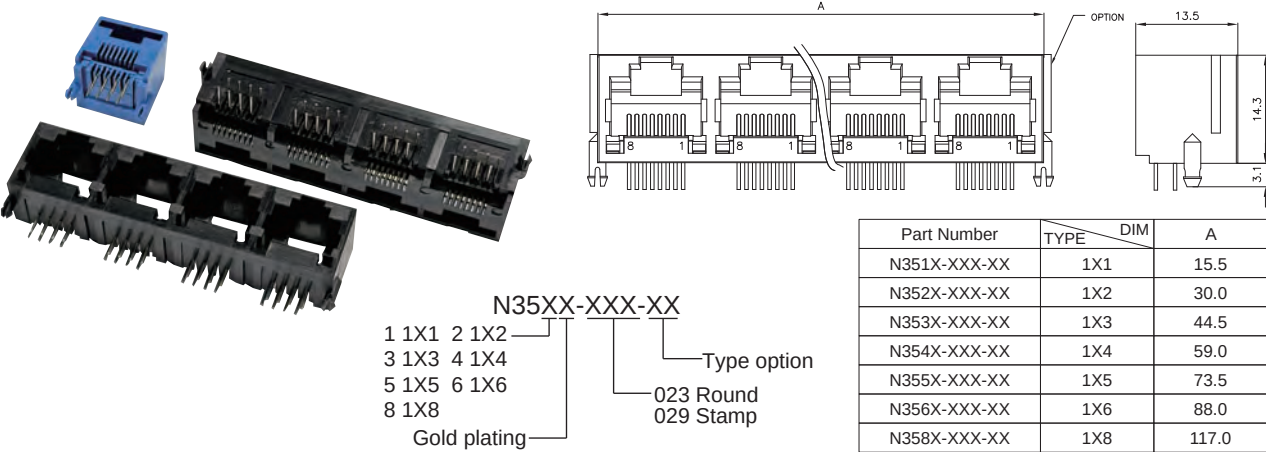
Side Entry 1XN Mini L/P 8P PCB Jack
