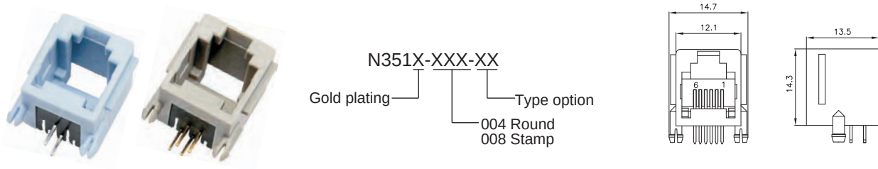
Side Entry 1XN Mini L/P 8P PCB Jack
